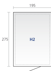
Afb. grootte H2. Standaarddeur kan vanaf grootte H2 in iedere zijwand worden ingebouwd.
